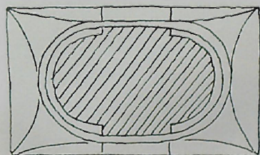
Сл. 17. Коњух, црква, мено с капителом и базом; шрафирано висина и дебљина зида и плоча у затвореним интерколумнијама.
