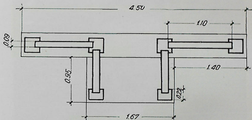
Сл. 28. Коњух, црква, основа олтарске преграде. Konjuh, église: plan de la cloison du sanctuaire
