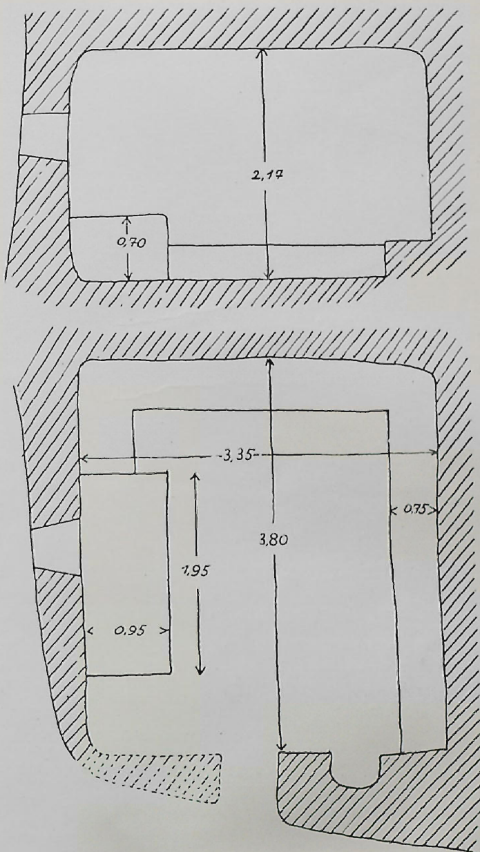
Сл. 4. Коњух, врх Големог Градишта, основа и пресек једне испоснице. Konjuh, sommet de Golemo Gradište, plan et coupe d'une cellule.
