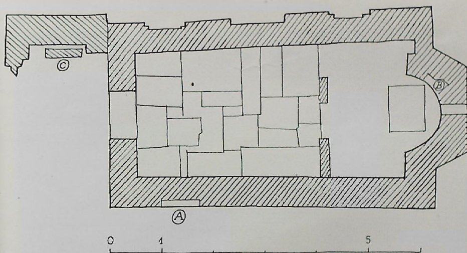
Сл. 7. Коњух, Црква св. Арханђела, основа. А. — латински натпис; В. — фрагмент скулптуре из VI в.; С. — старосрпска надгробна плоча. Konjuh, église du saint Archange, plan. A. — Inscription latine. B. — Fragment de sculpture du VI e siècle. C. — Dalle funéraire ancienne serbe.
